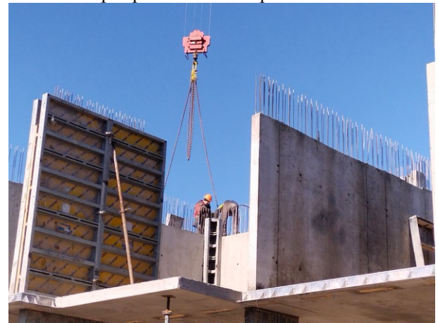
Установка опалубки для бетонирования стен второго этажа
